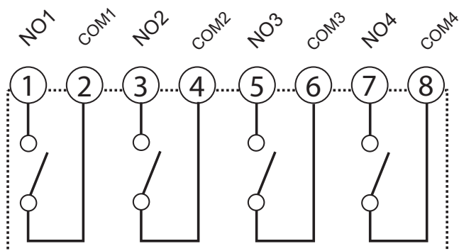
Fig. 27 MF I6 R4. 4 salidas de relé
