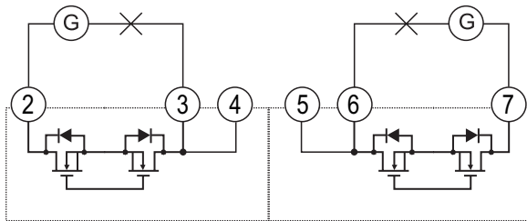
Fig. 19 MO O2. Salida opto-mosfet estática doble.
