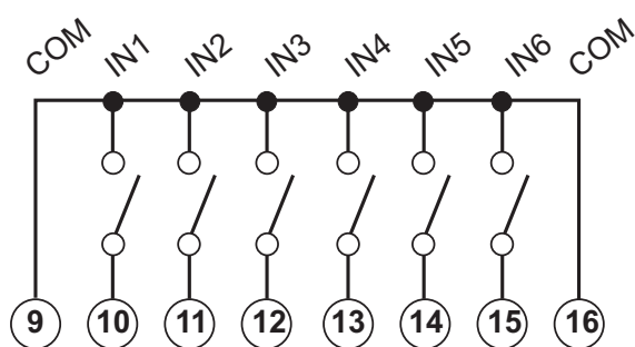
Fig. 26 MF I6 R4. 6 entradas digitales
