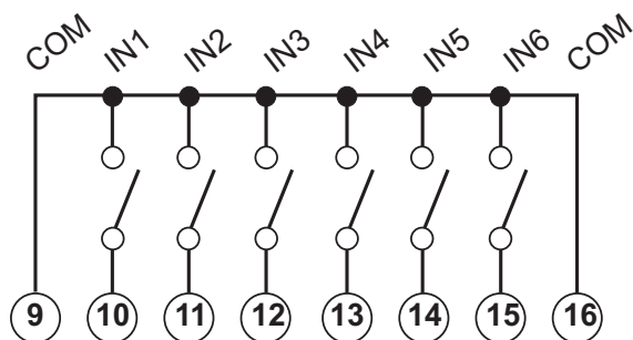
Fig. 24 MF I6 O6. 6 entradas digitales
