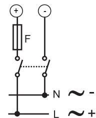
Fig. 17 Alimentación auxiliar (H). Fusible 250 V [T] 630 mA (F). Alimentación auxiliar (L). Fusible 250 V [T] 630 mA (F).
