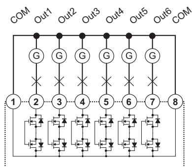
Fig. 25 MF I6 O6. 6 salidas estáticas
